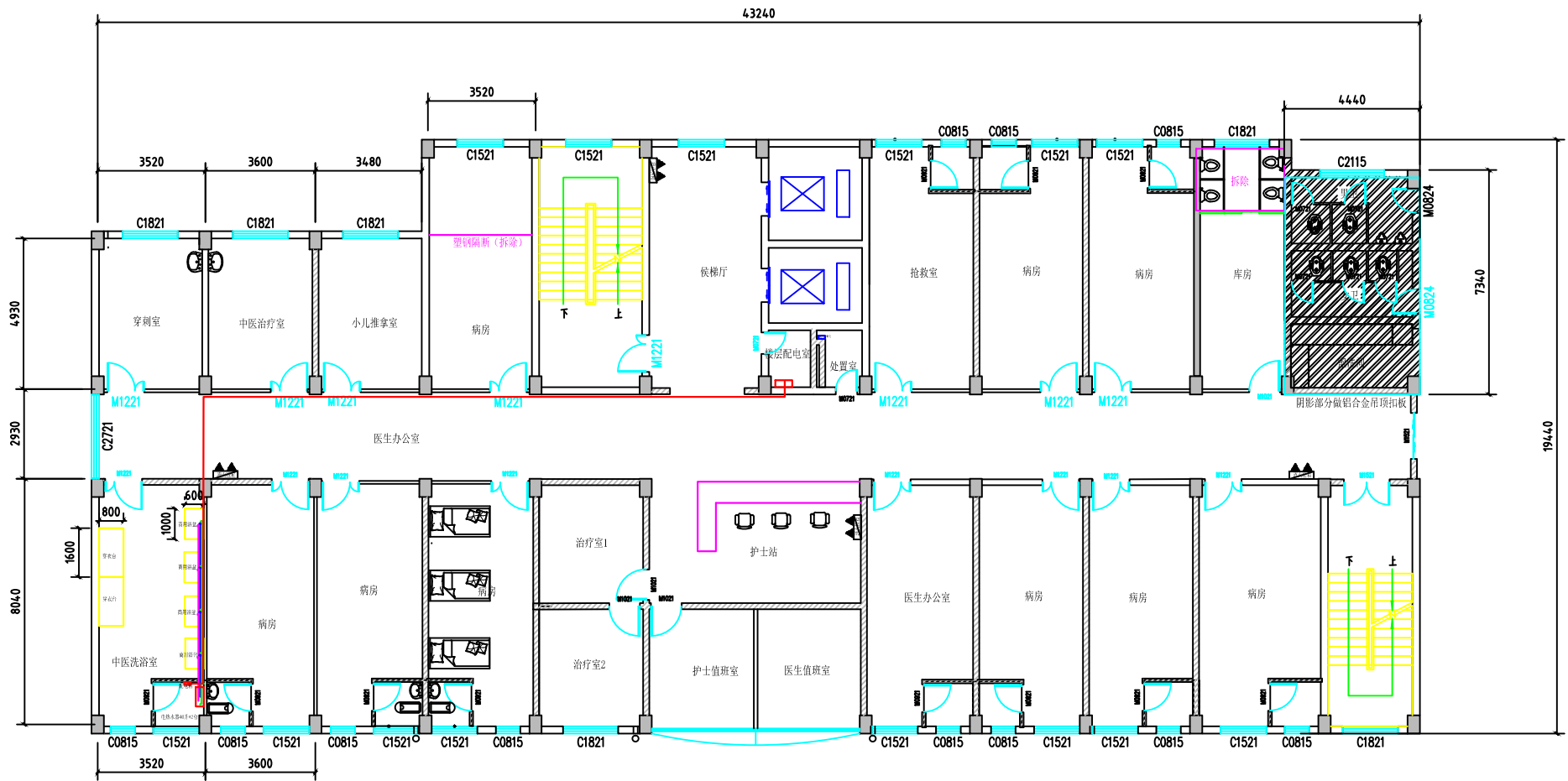
住院楼5层儿科改造示意图 1:100
