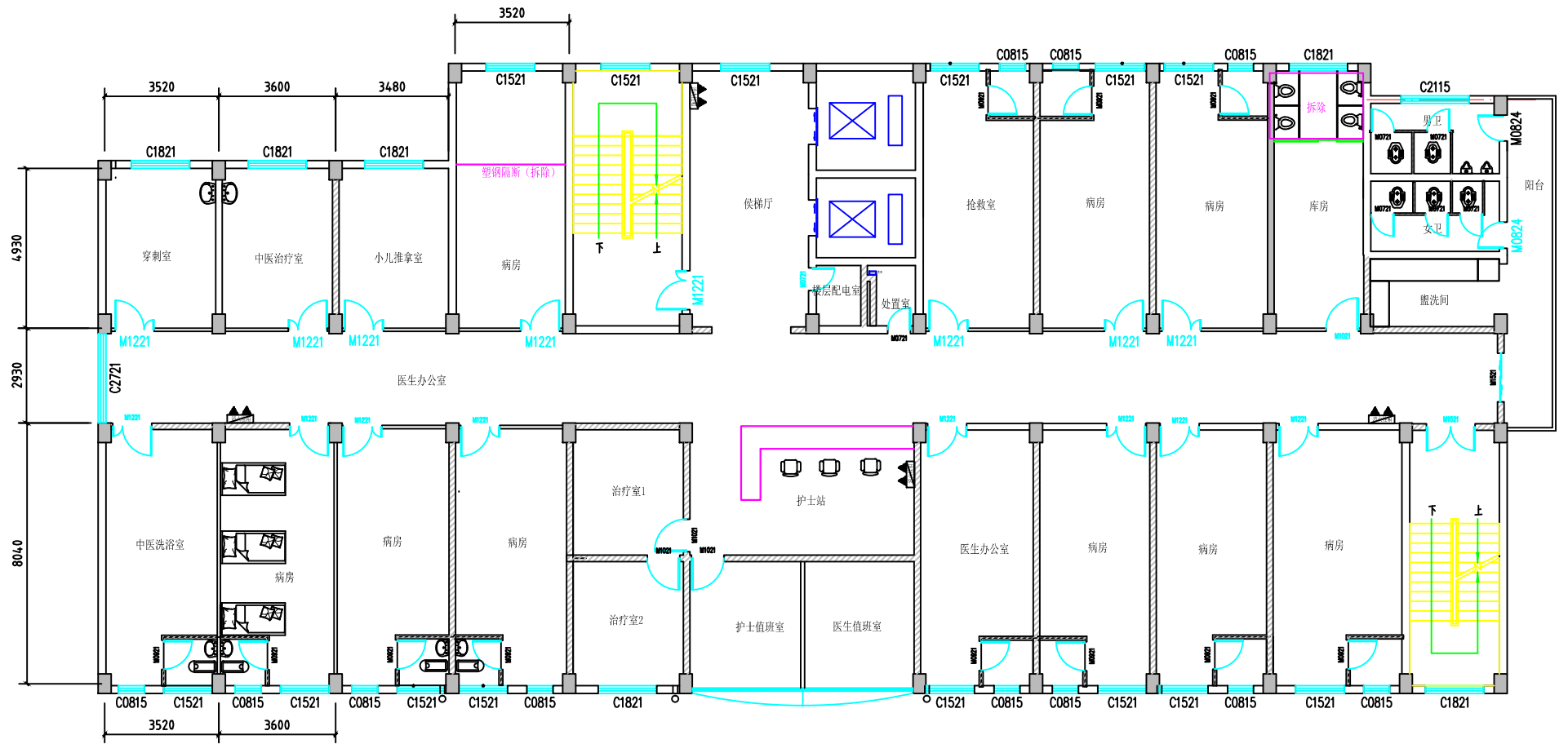
住院楼5层平面示意图 1:100
